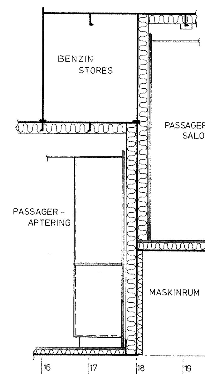
SNIT M-M
