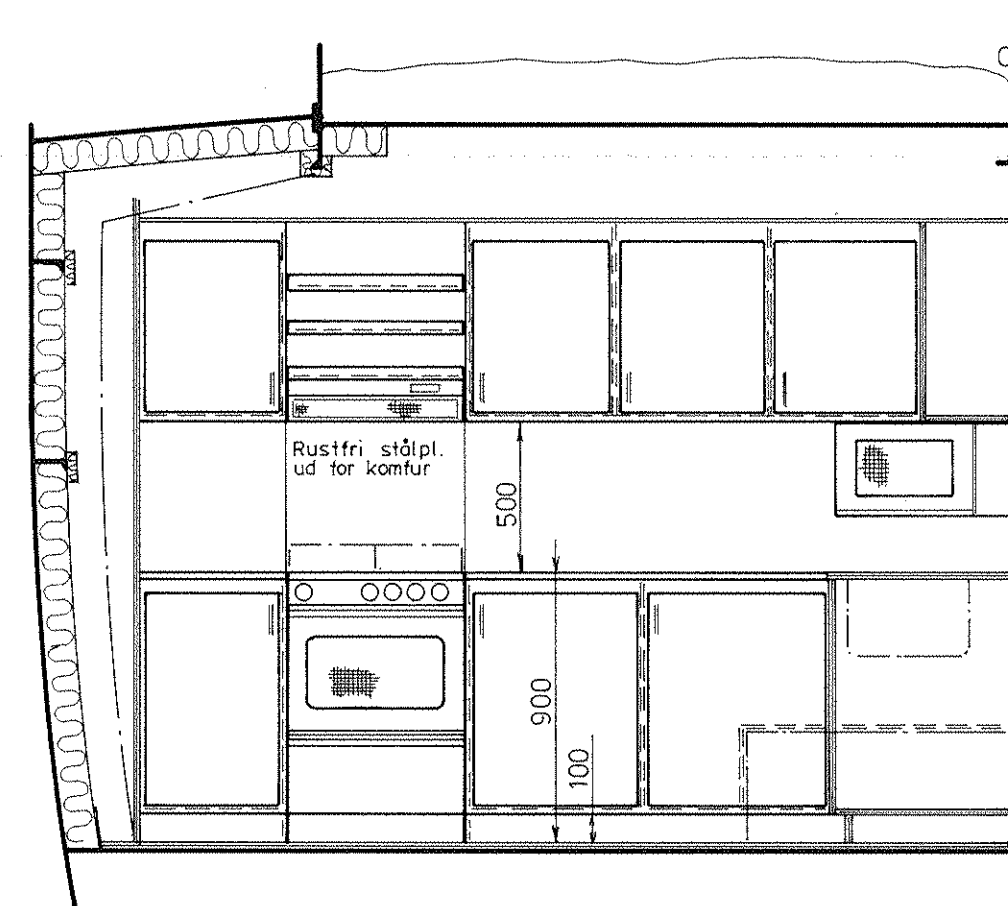
SNIT G-G
