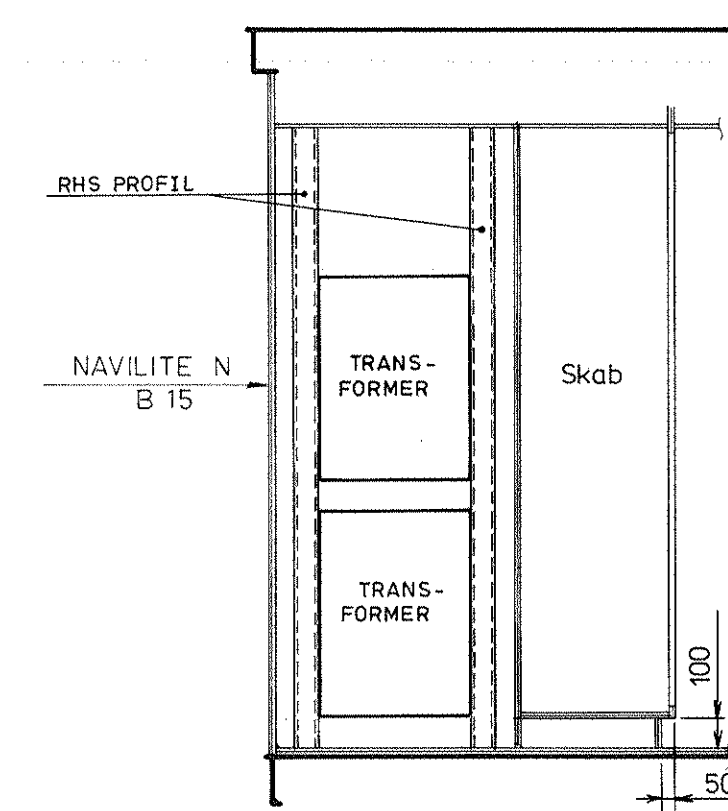
SNIT I-I
