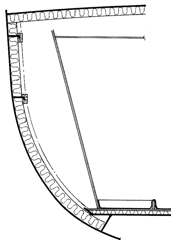
SNIT C-C
