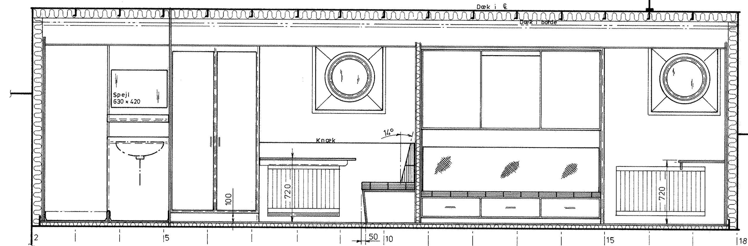
SNIT C-C
