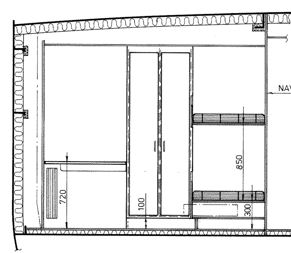
SNIT M-M
