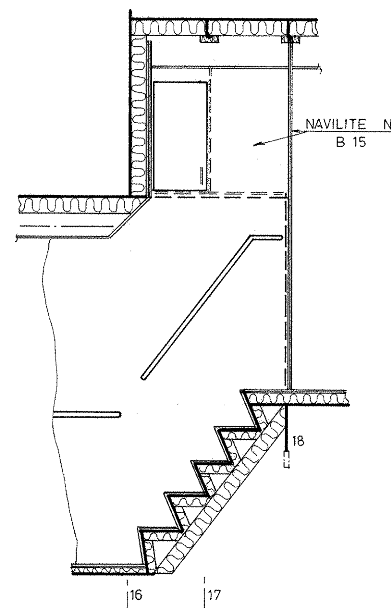
SNIT L-L
