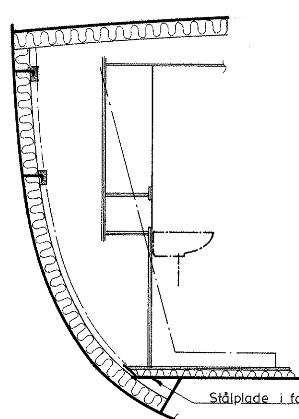
SNIT D-D
