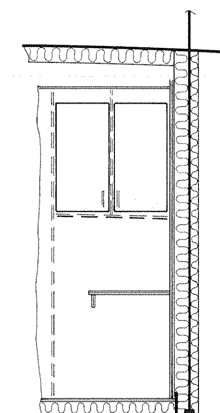
SNIT D-D
